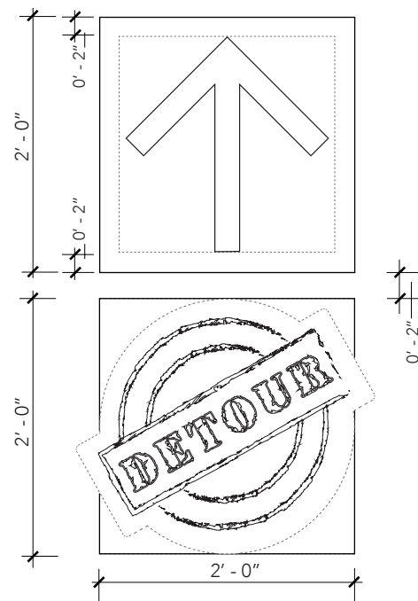
1 PLAN SCALE: 3/4" = 1' - 0"
