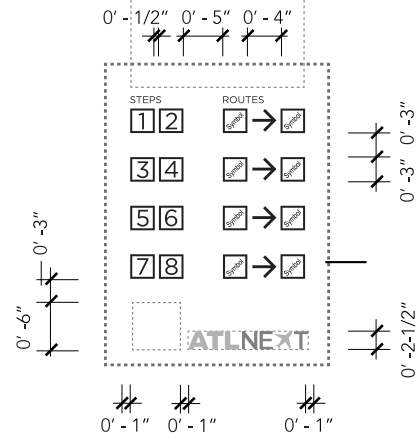
3 FRONT SCALE: 1/2" = 1' - 0"
