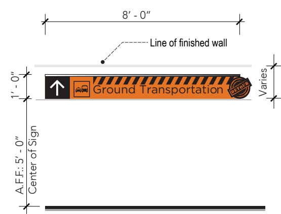
8 ELEVATION (WALL) SCALE: 1/2" = 1' - 0"
