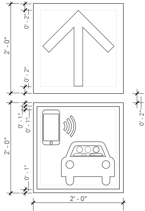
1 PLAN SCALE: 3/4" = 1' - 0"
