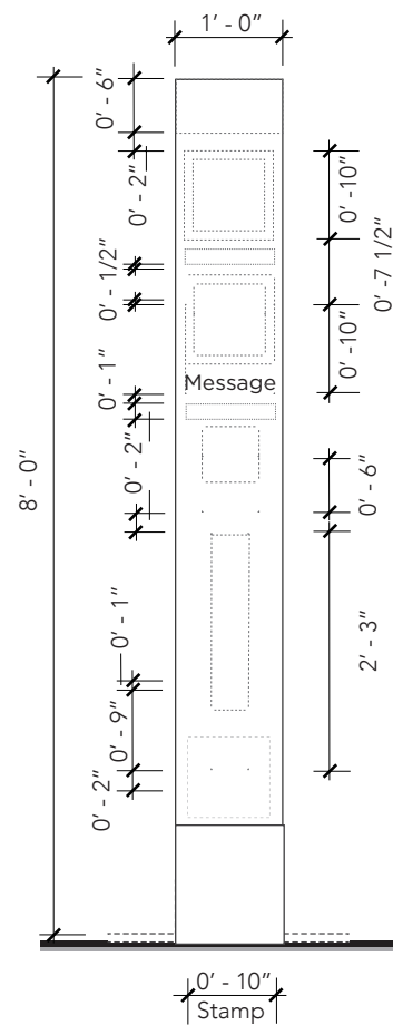
6 FRONT - SIDE B SCALE: 1/2" = 1' - 0"
