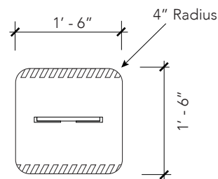
1 PLAN SCALE: 1/2" = 1' - 0"
