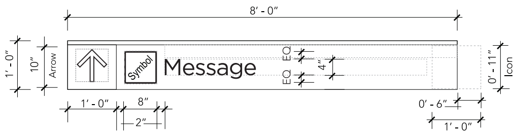
2 FRONT SCALE: 1/2" = 1' - 0"
