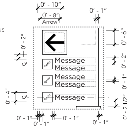
3 DETAIL SCALE: 1/2" = 1' - 0"
