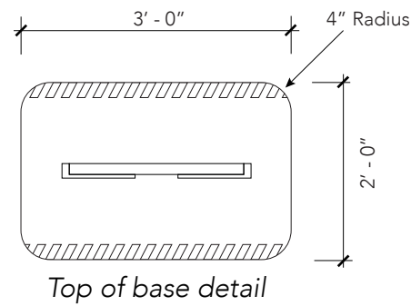
1 PLAN SCALE: 1/2" = 1' - 0"
