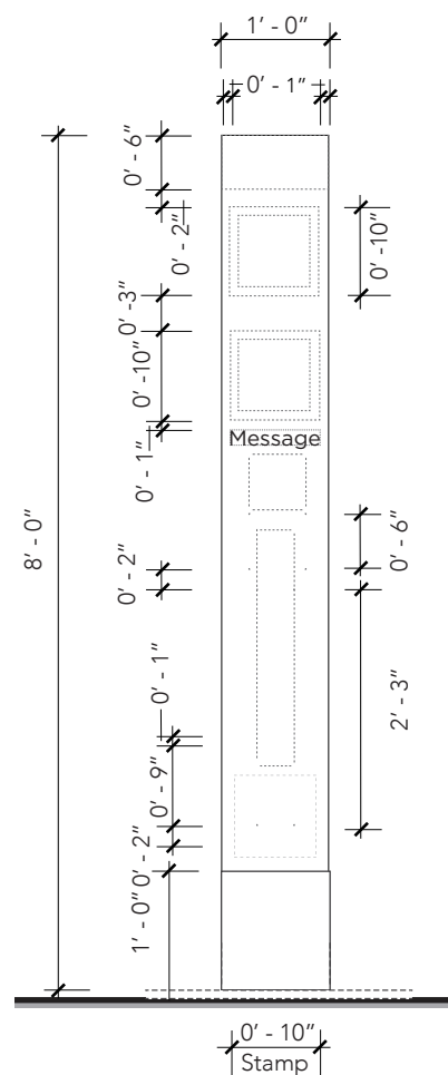
2 FRONT - SIDE A SCALE: 1/2" = 1' - 0"
